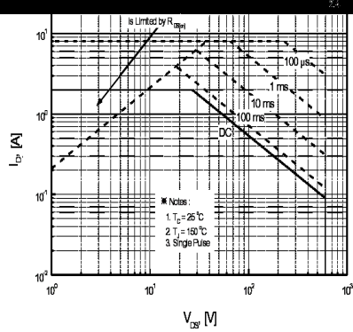
I_D - V_{DS}
