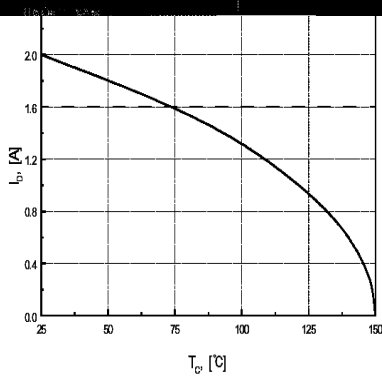
I_D - T_J
